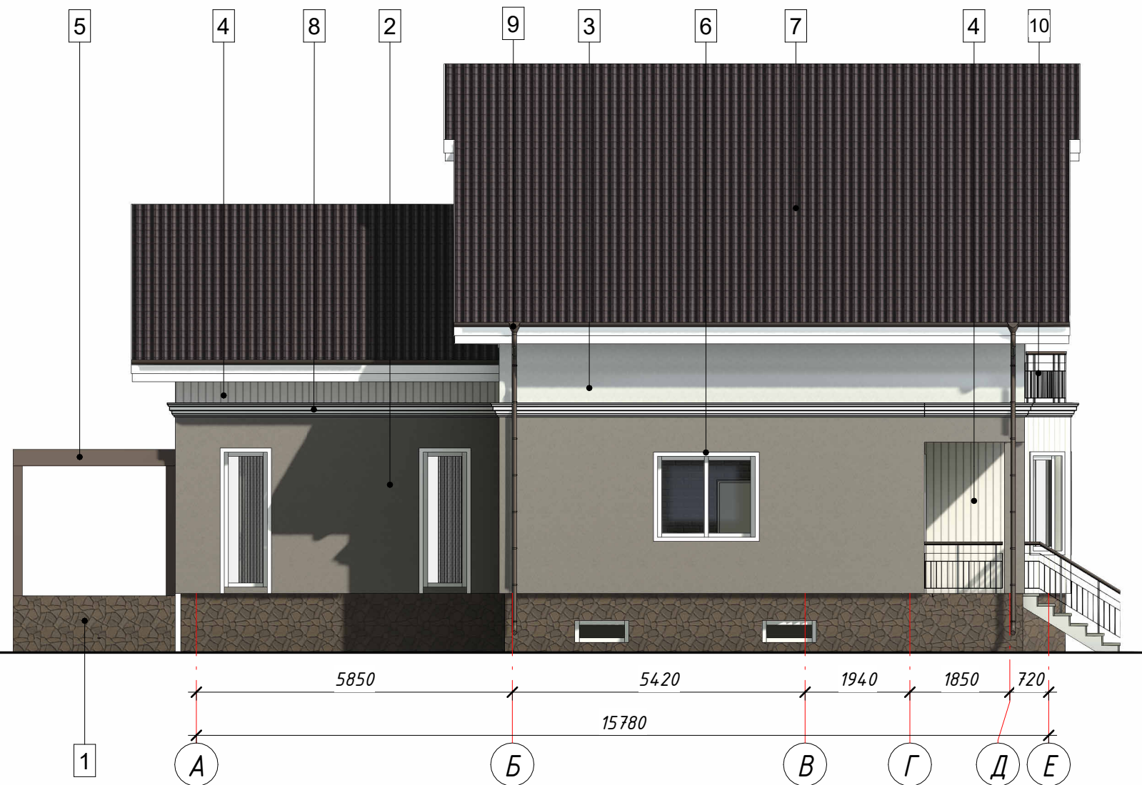
Фасад в осях А-Е
