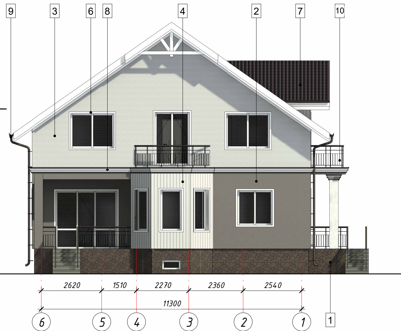
Фасад в осях б-1
